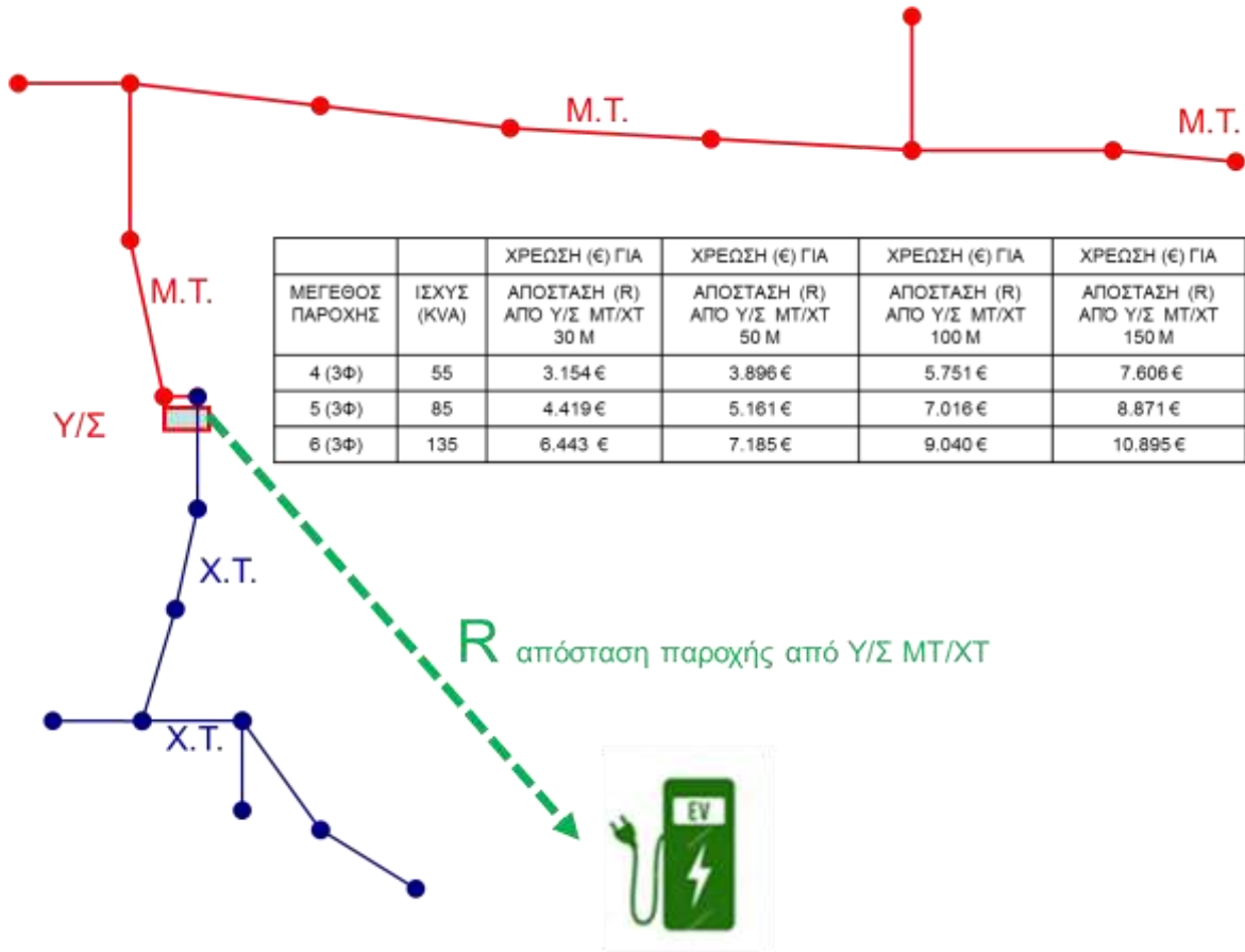
Σχήμα 2: Ενδεικτικά παραδείγματα υπολογισμού κόστους σύνδεσης για αποστάσεις <30m , 50m , 150m από τον πλησιέστερο Υ/Σ ΜΤ/ΧΤ
